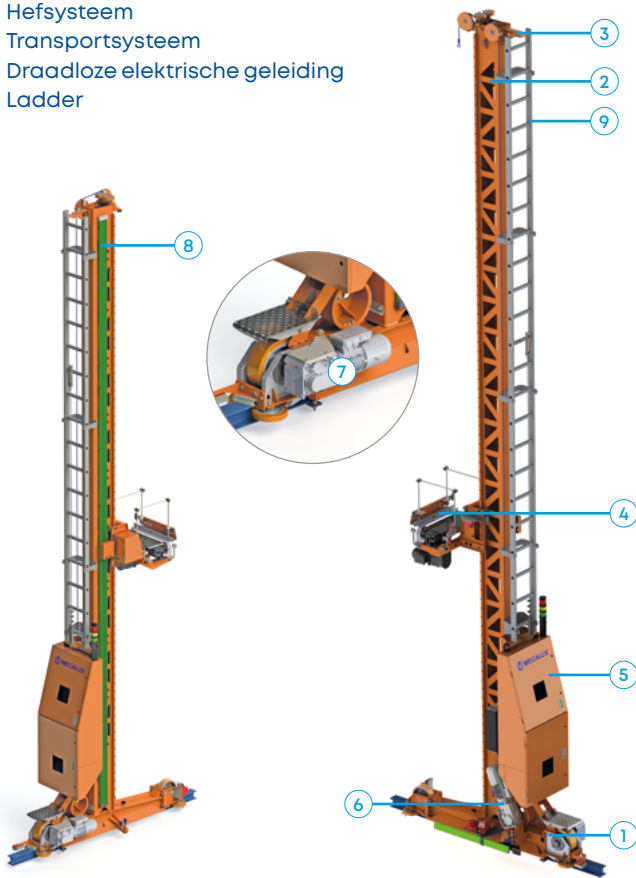
ML50-stapelkraan met enkele mast Verwerkt dozen tot 50 kg op hoogtes tot 9 m.
